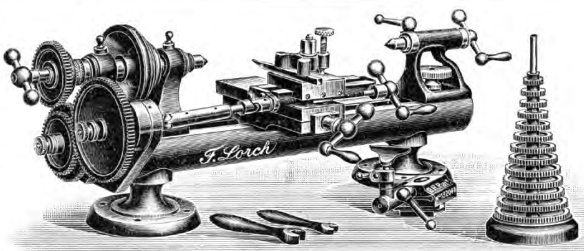
No. 6734. Abbildung zeigt den Patent-Drehstuhl „LL“ No. 1 auf 2 niedrigen Füßchen, mit Kreuzsupport No. 5 und der Gewindeschneidanordnung, einschließlich 16 gefräster Rotgußräder No. 1b. Komplette M. 262.50
